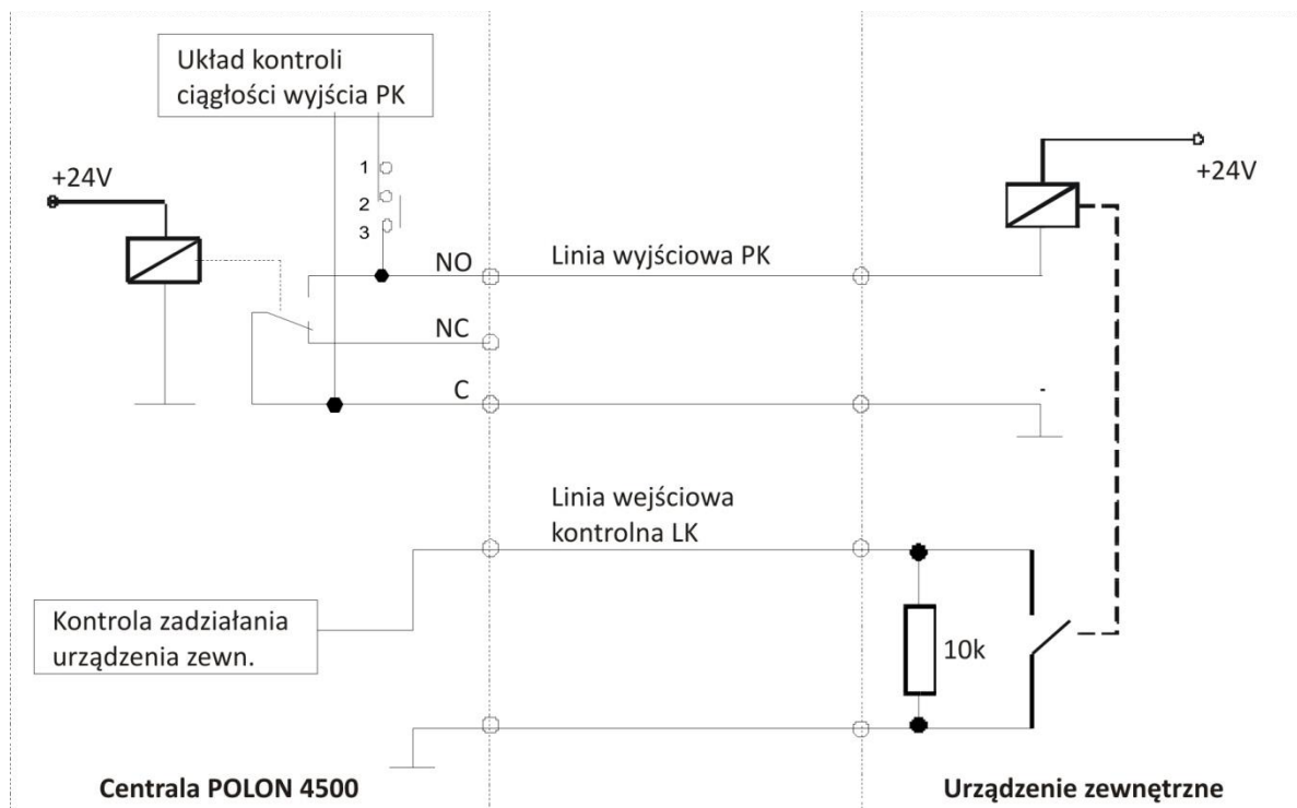
Rys. 5.5 Przykładowe wykorzystanie linii kontrolnej przypisanej do wyjścia przełącznikowego
