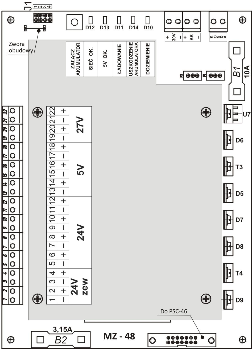
Rys. 5.11 Moduł zasilania centrali MZ-48.
