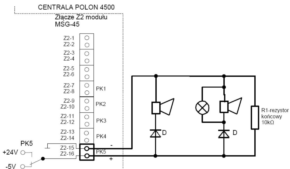
Rys. 9.15 Przykład połączenia wyjścia potencjałowego.
