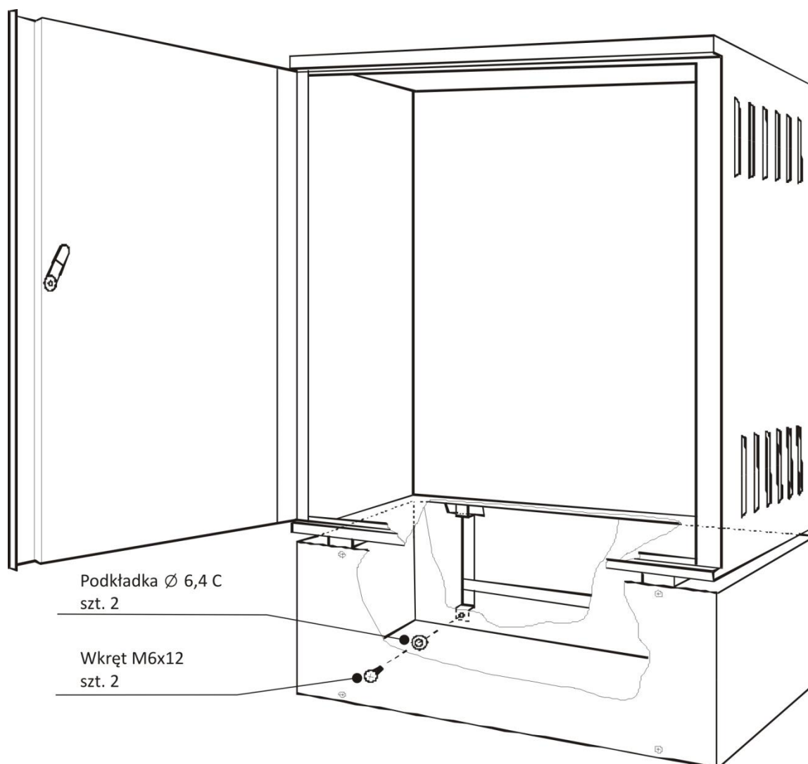
Rys. 15.2 Mocowanie pojemnika akumulatorów PAR-4800
