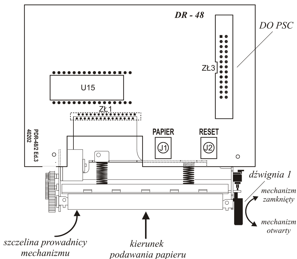
Rys. 5.10 Widok drukarki DR-48 od strony wnętrza centrali
